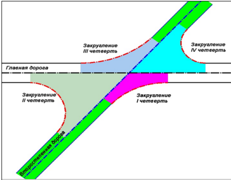
Схема пересечения от оси главной дороги
