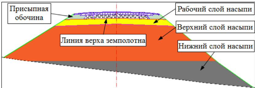
Рабочий слой насыпи
