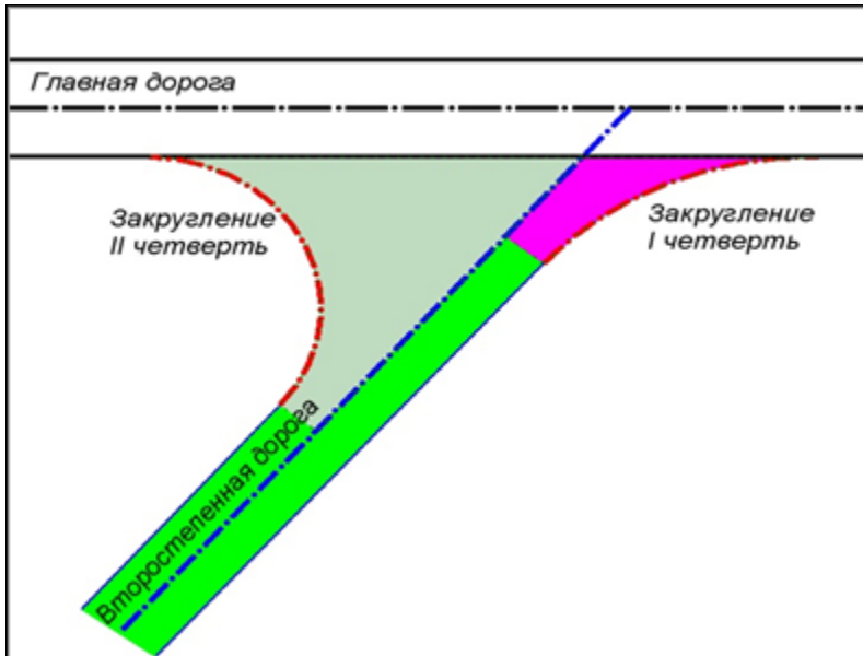
Схема примыкания от кромки главной дороги
