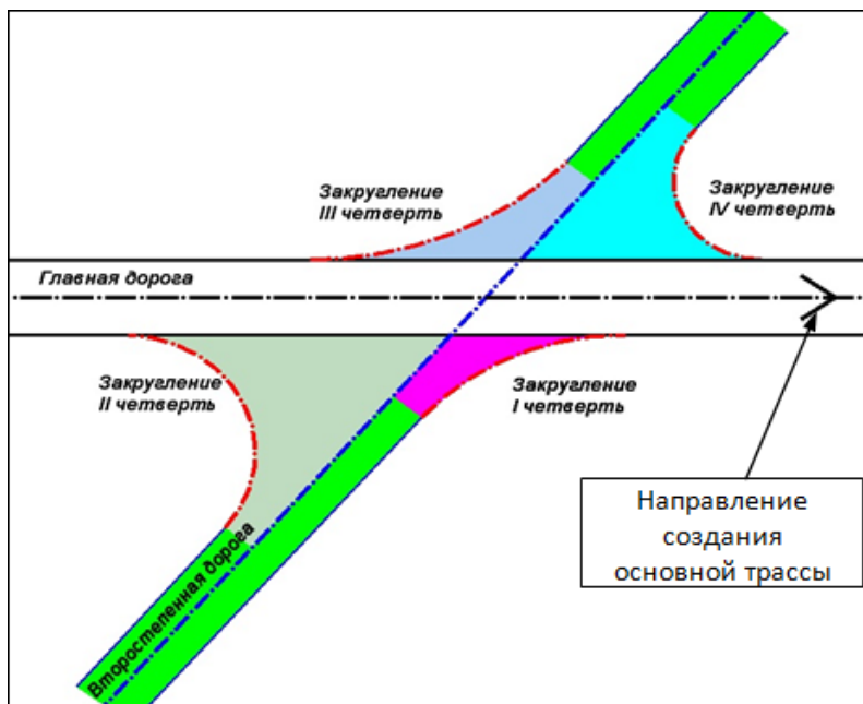
Схема примыкания от оси главной дороги
