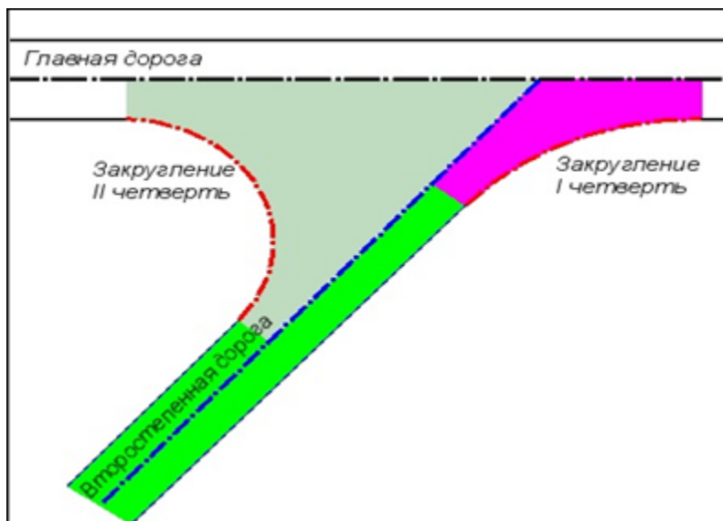
Схема примыкания от оси главной дороги
