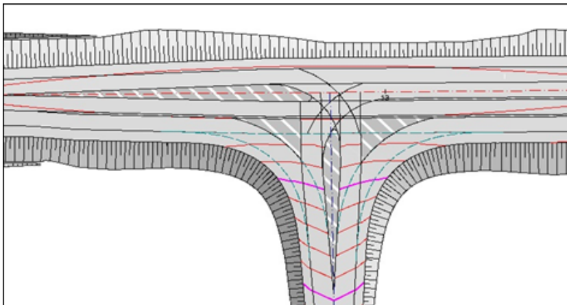
Пример канализированного примыкания
